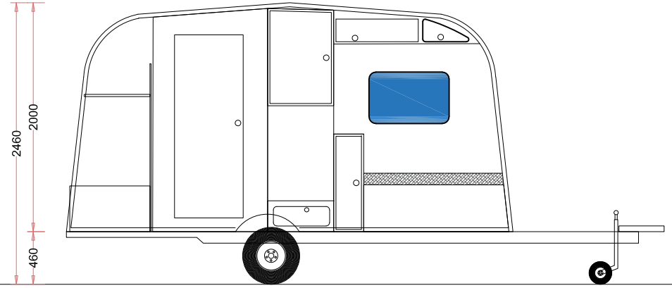
BOYUNA KESİTİ
