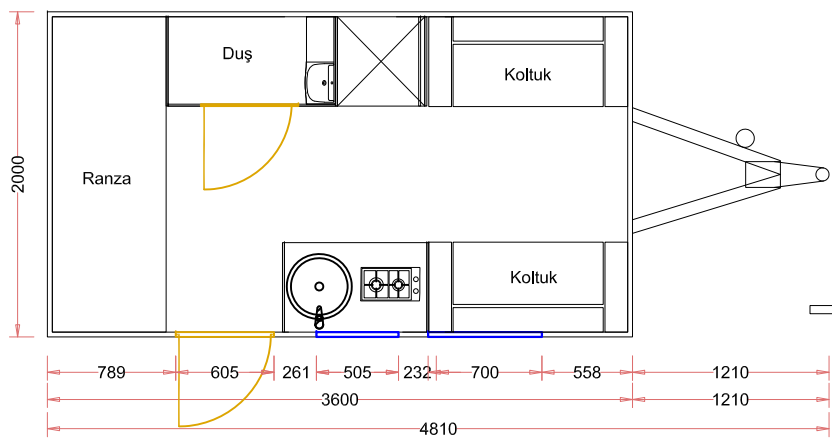
GİRİŞ KATI PLANI
